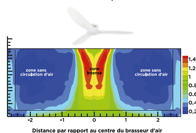
Brasseur d'air à pales
